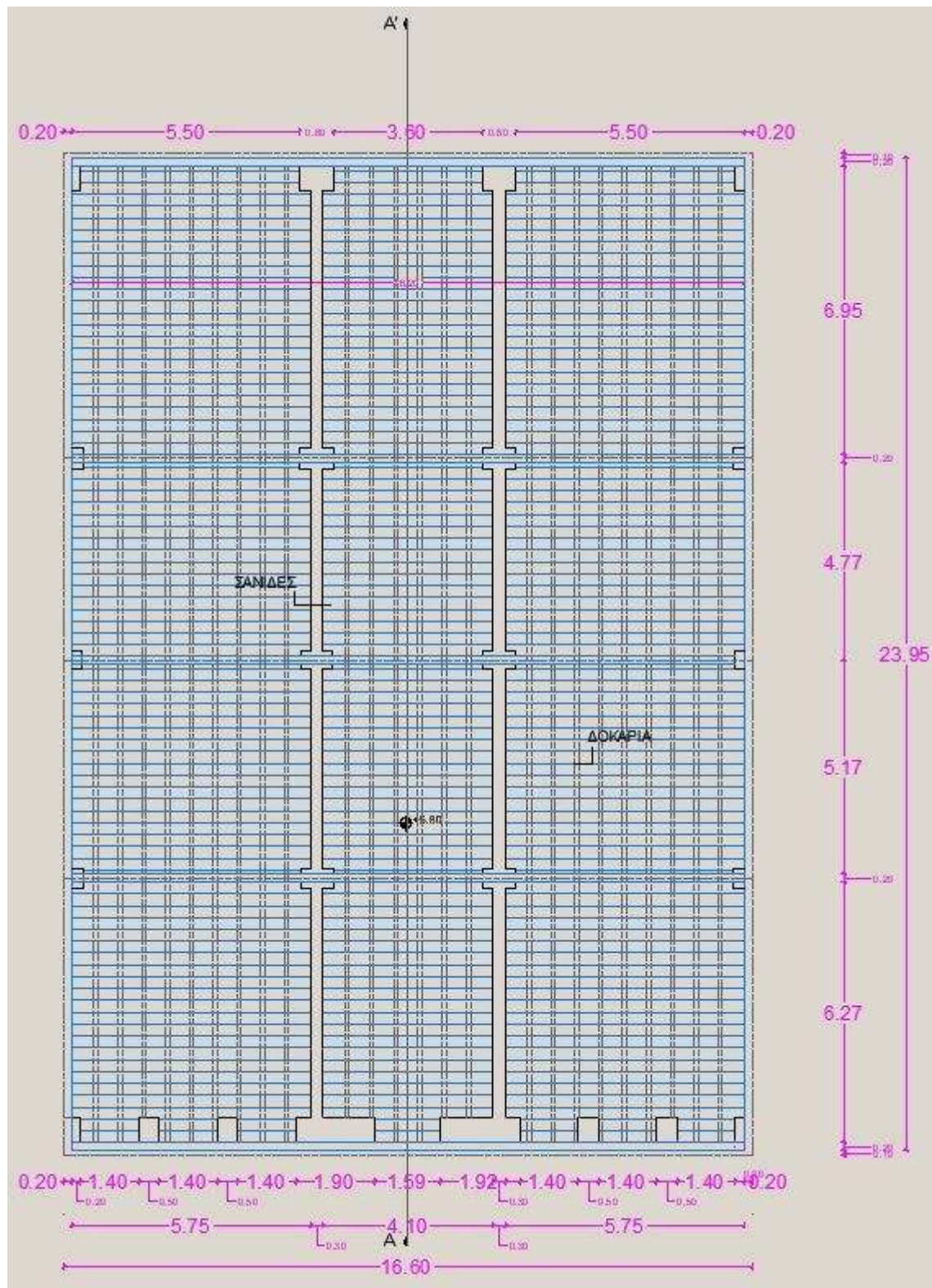
Εικόνα Ι.6. Κάτοψη Έδρασης Στέγης
