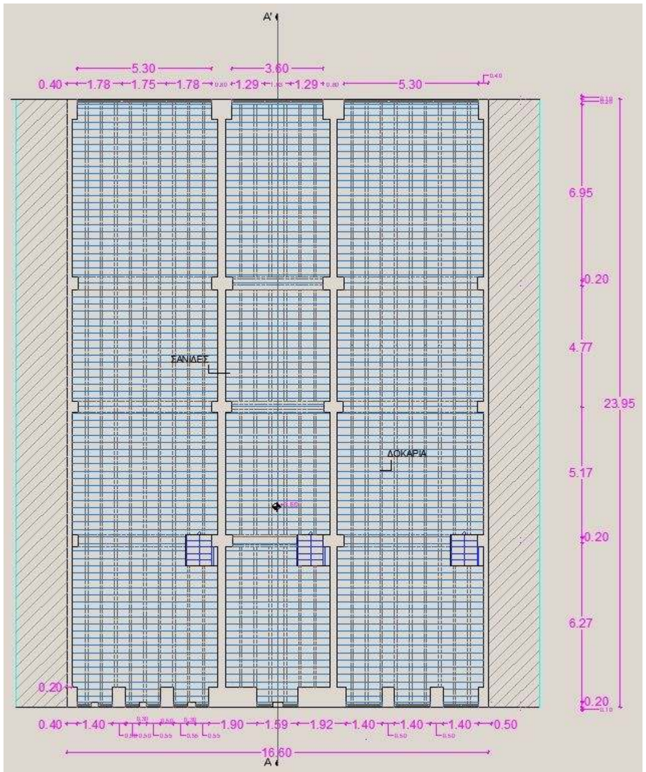
Εικόνα Ι.5. Κάτοψη Παταριού
